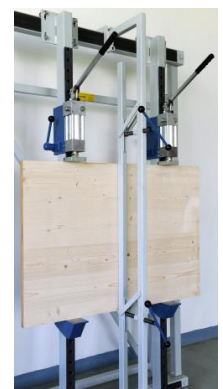
Bündighalter
